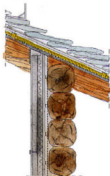
R ascard originale, costruzione a blockbau, restaurato e rimontato - dettaglio incastro-ballatoio
